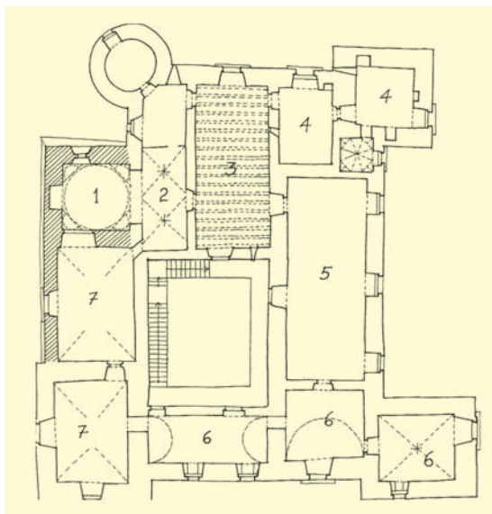
Fig. A - Ipotesi di restituzione del piano nobile del castello al secolo XVI, con l'ampliamento realizzato tra il 1573 e il 1584 (a tratteggio): (1) Cappella cinquecentesca, (2) Anticappella (già cappella prima del 1574 ?), (3) Salone del castello con le capriate lignee del '400 dipinte probabilmente nel '600, (4) Quarto di don Cesare , (5) Sala d'armi ?, (6) Appartamento delle marchese di Geraci, (7) Appartamento dei marchesi di Geraci ? (Da E. Magnano di San Lio, Castelbuono capitale dei Ventimiglia cit. , p. 101).
